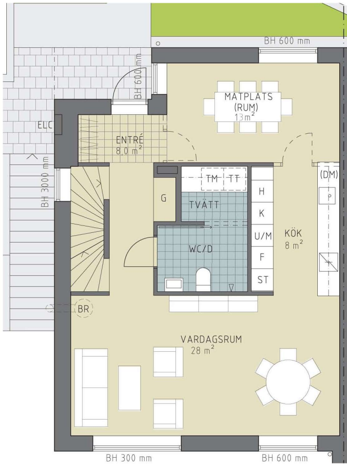
ENTRÉPLAN
