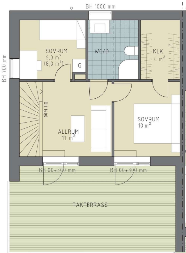
ÖVRE PLAN
