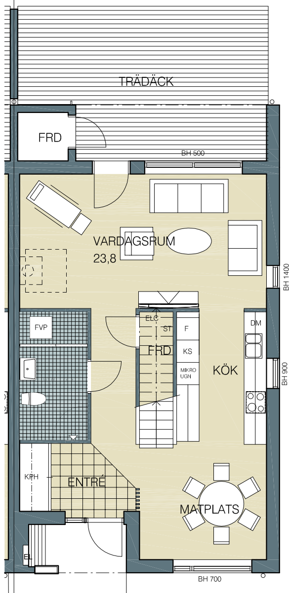
ENTRÉPLAN
