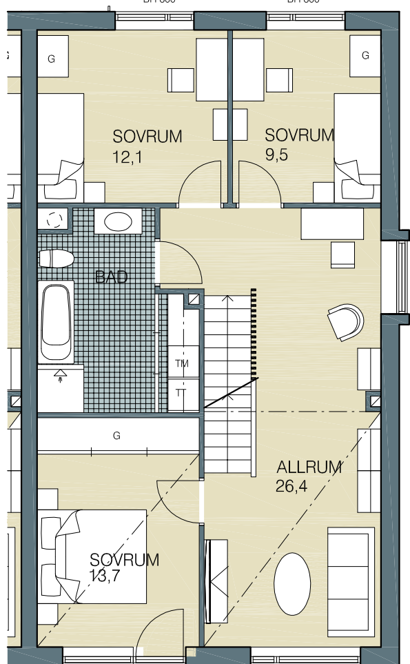
ÖVRE PLAN
