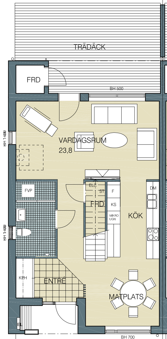
ENTRÉPLAN
