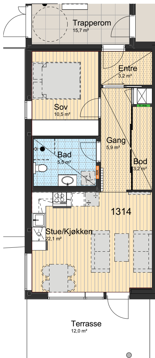
1:100 Plan 3.etasje
