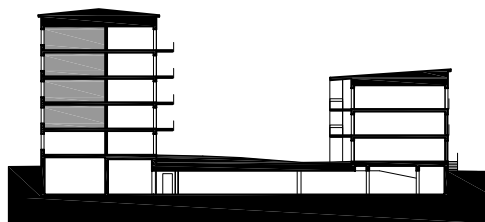
SEKTION D-D
