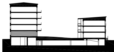
SEKTION D-D
